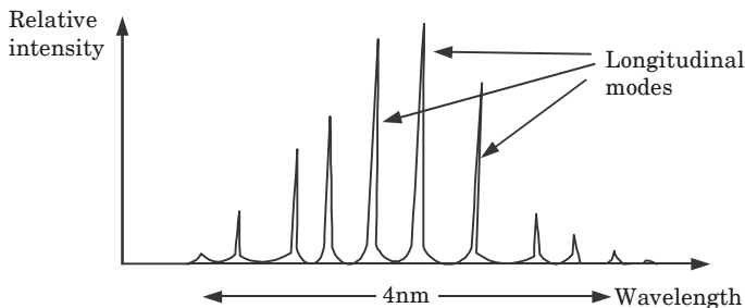
Fig. 3.18.1. Laser modes.
