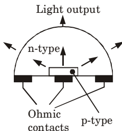
Fig. 3.4.2. Dome LED.
